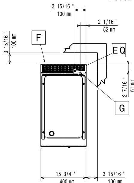
Boven aanzicht
