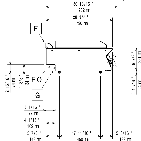
Zij aanzicht
